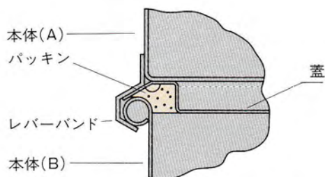
LBF 24~47 積み重ね図
