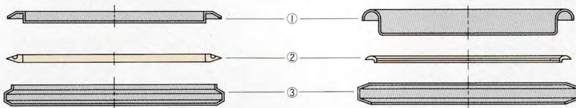
LBF 24~47 L型パッキン使用
