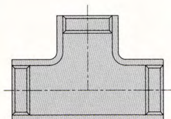
ねじ込みチーズ
