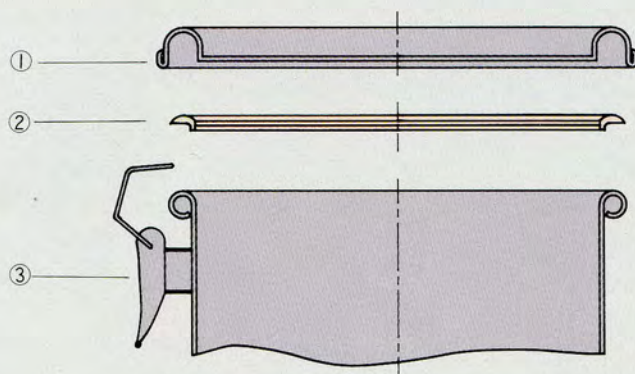
キャッチクリップ式密閉蓋
