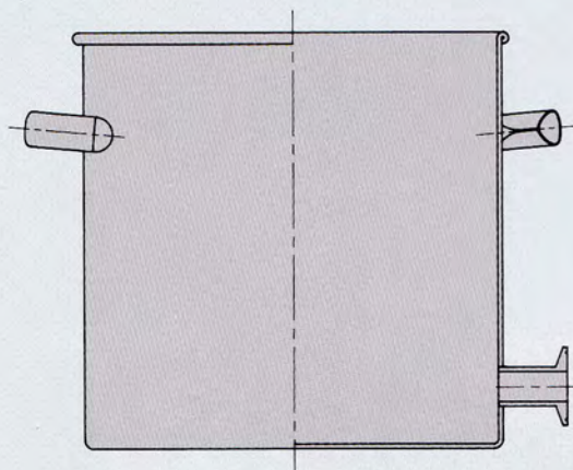
加工例 2
