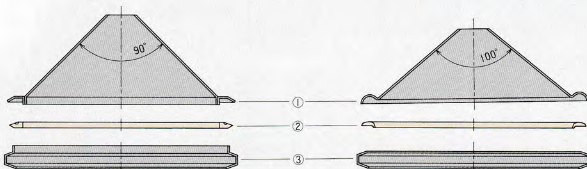
HTL 24~47 L型パッキン使用
