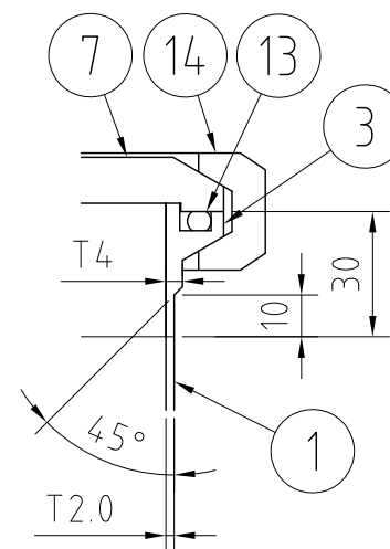
B部詳細 S=1:2
