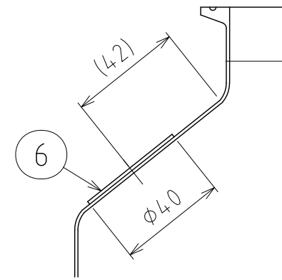
B-B 当て板詳細 S=1:2
