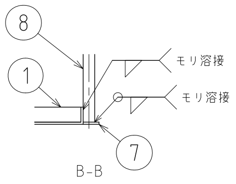
パイプハンドル取付部詳細
