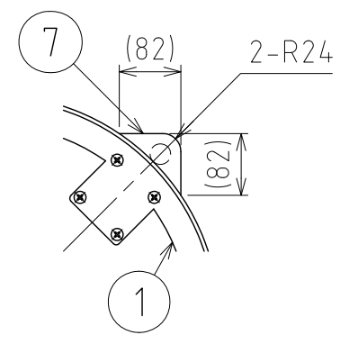
パイプハンドル取付座詳細
