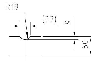
袴切り欠き詳細図
