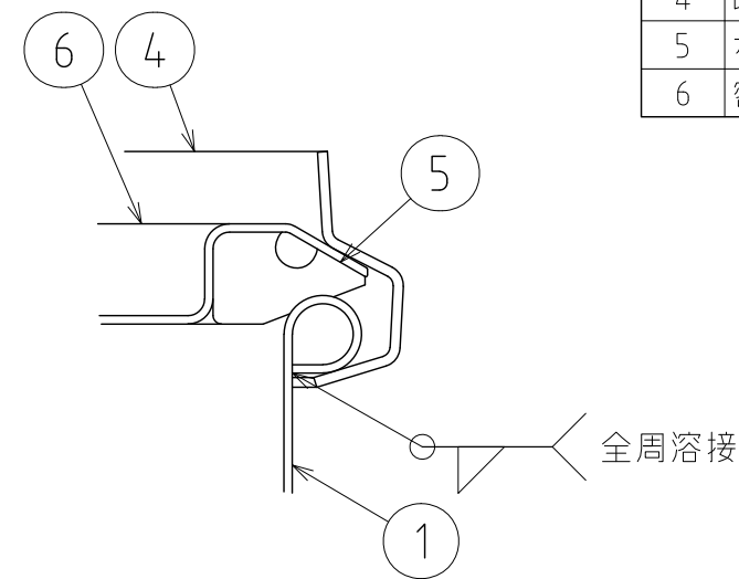
B部詳細 S=1:1
