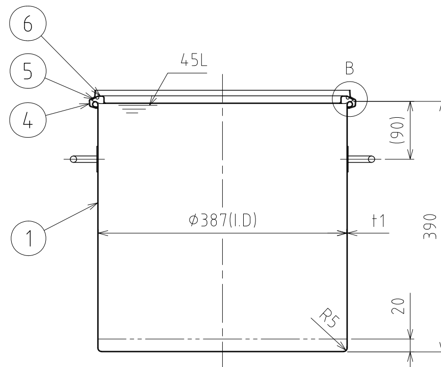
A-A
