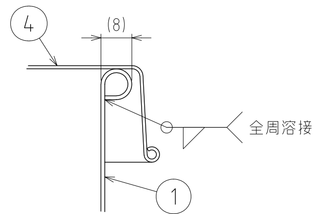
B部詳細 S=1:1
