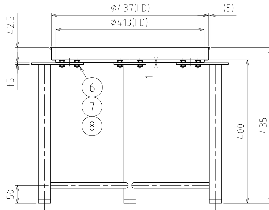
A-A
