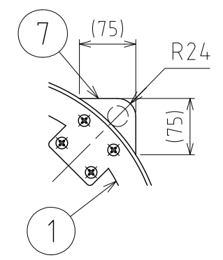
パイプハンドル取付座詳細
