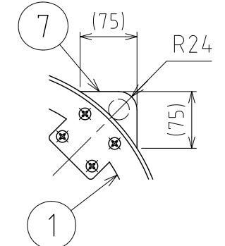
パイプハンドル取付座詳細
