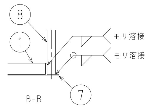
パイプハンドル取付部詳細
