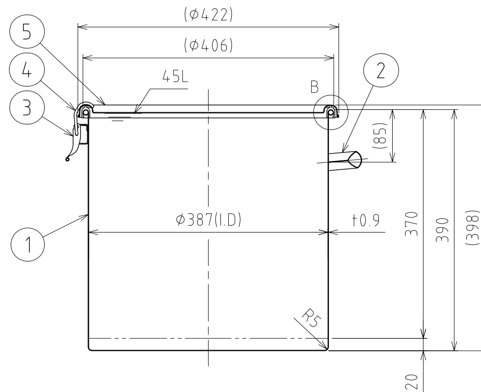
A-A
