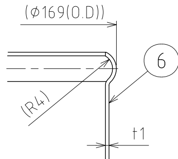
C部詳細 S=1:1
