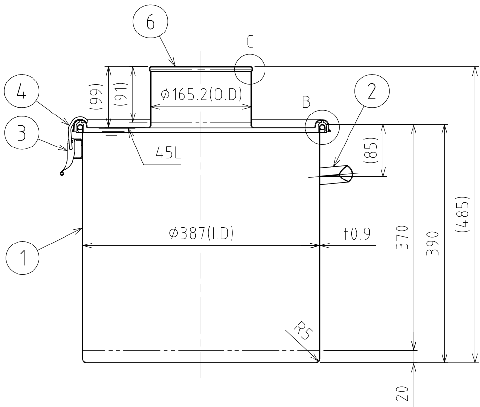
A-A
