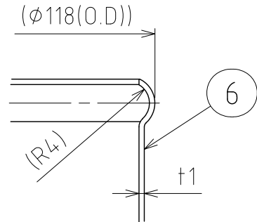
C部詳細 S=1:1
