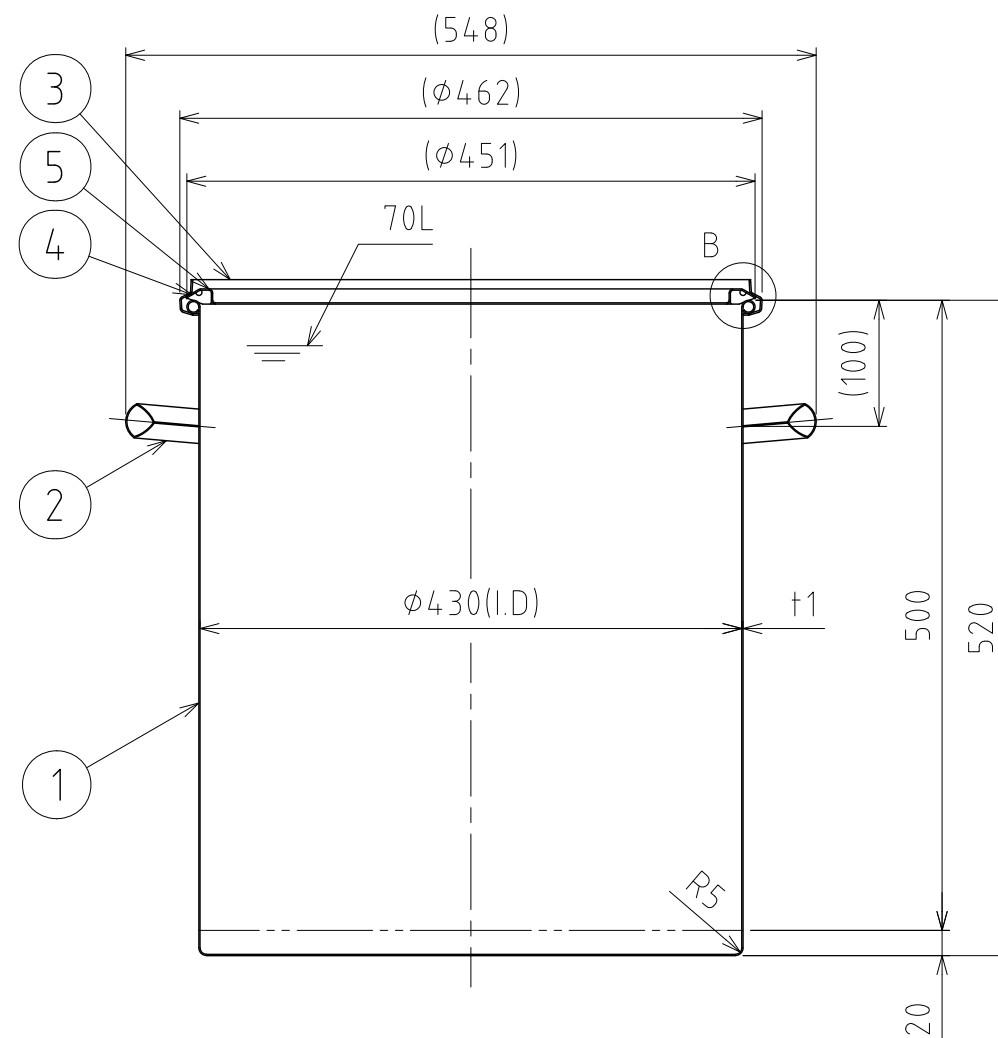
A-A
