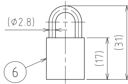
南京錠 S=1:1
