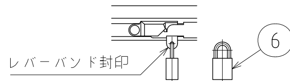
C部詳細 S=1:3
