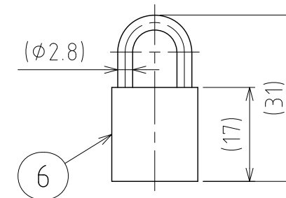
南京錠 S=1:1
