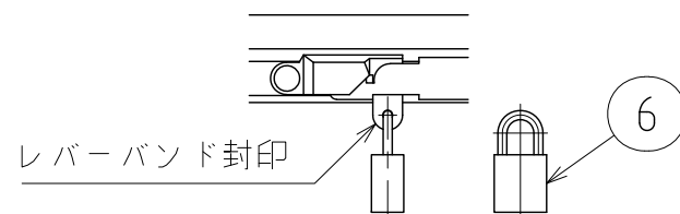
C部詳細 S=1:2.5
