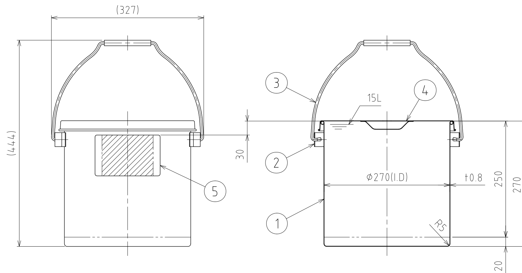
A-A
