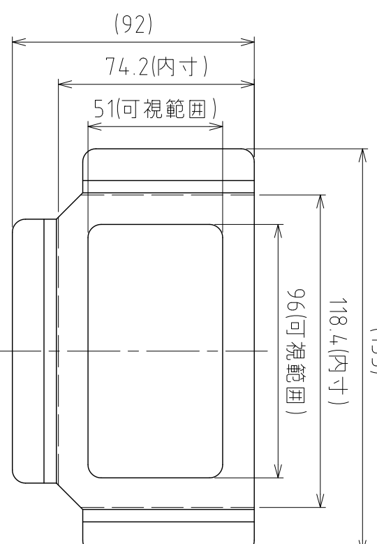
カードホルダー詳細 S=1:2
