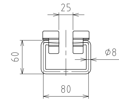
折りたたみ取っ手正面図
