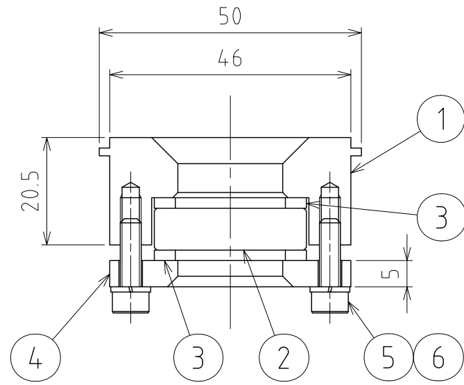
A部詳細 S=1:1 (断面図)
